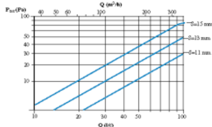
ÖV-C rektangulär lucka
