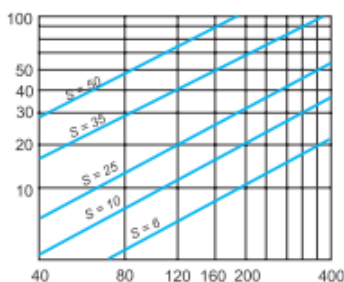
ÖV-A rektangulär lucka
