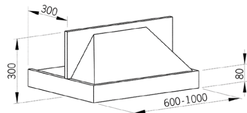
Måttskiss
