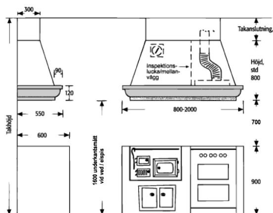
Måttskiss
